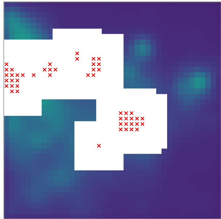
Scipy
